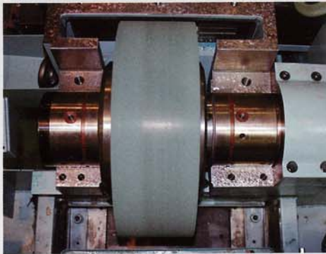
研削砥石スピンドルユニット
